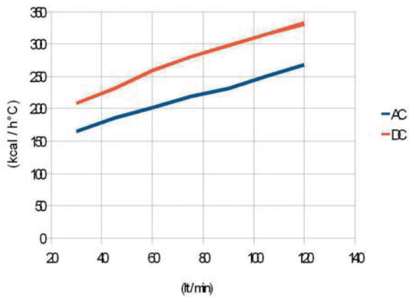
Leistungdiagramm/Performance Diagram
